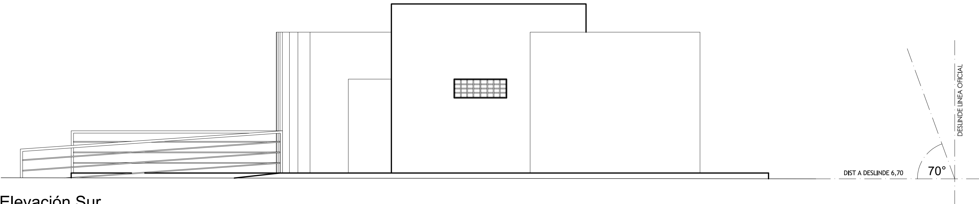
Camarines, Elevación Sur Esc. 1:500
