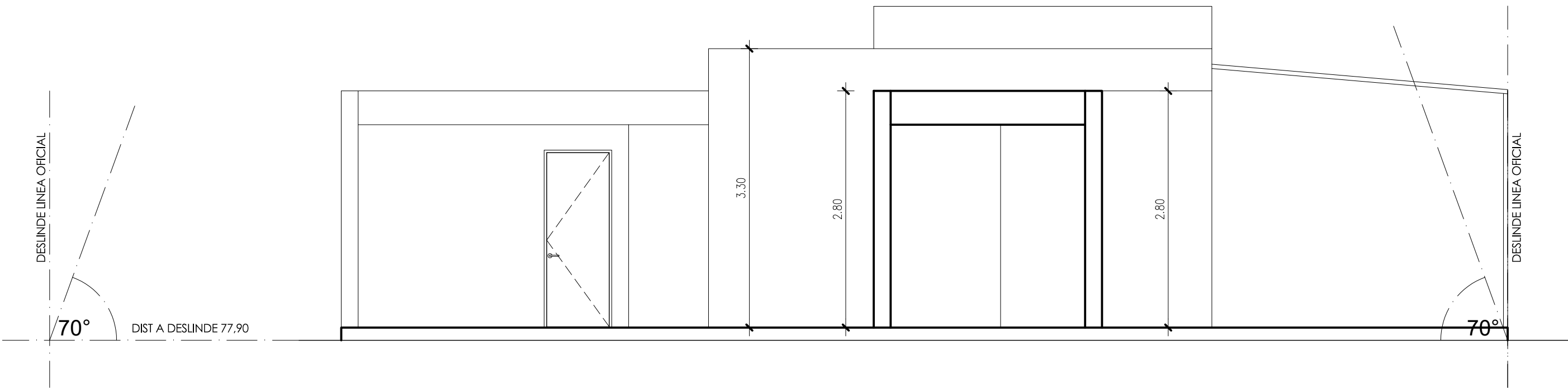
Kiosco / Enfermería, Elevación Oriente Esc. 1:50
