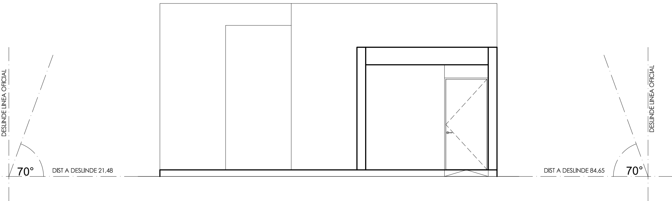
Acceso, Elevación Sur Esc. 1:50
