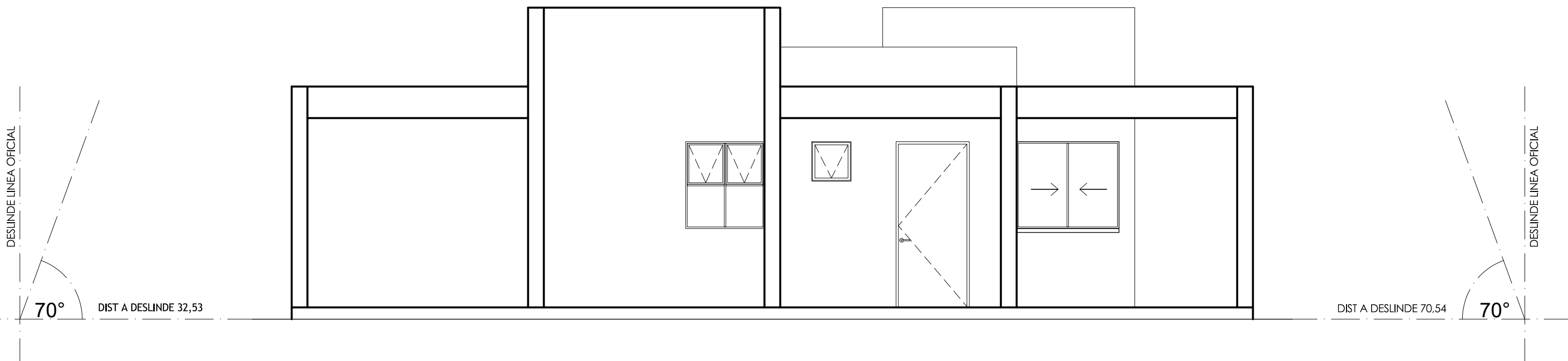
Acceso, Elevación Oriente Esc. 1:50
