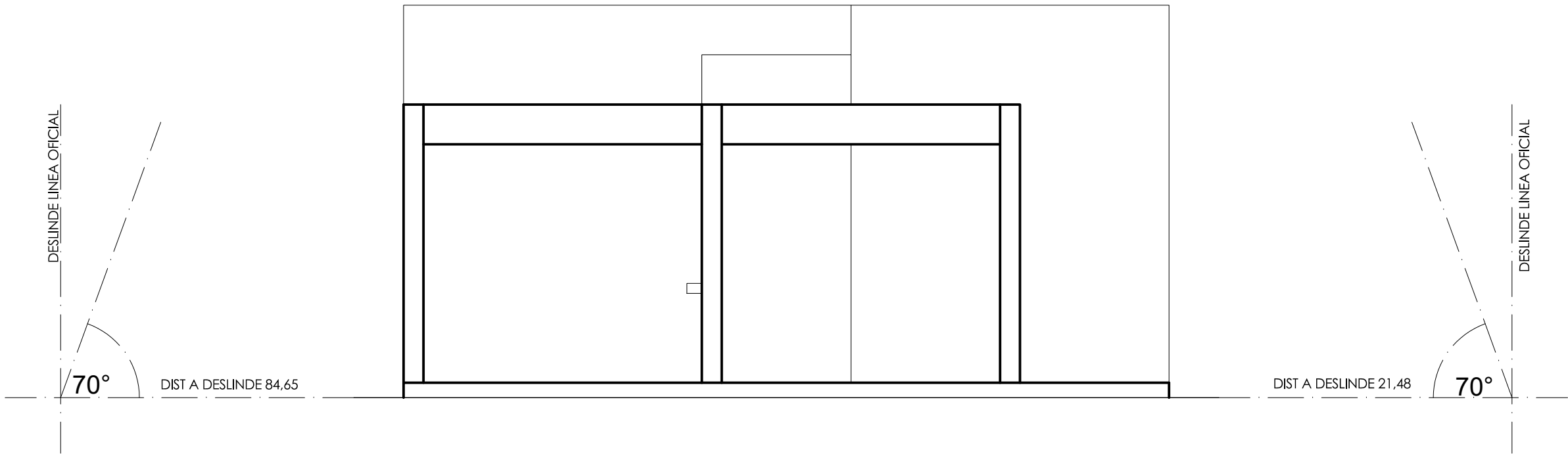
Acceso, Elevación Norte Esc. 1:50
