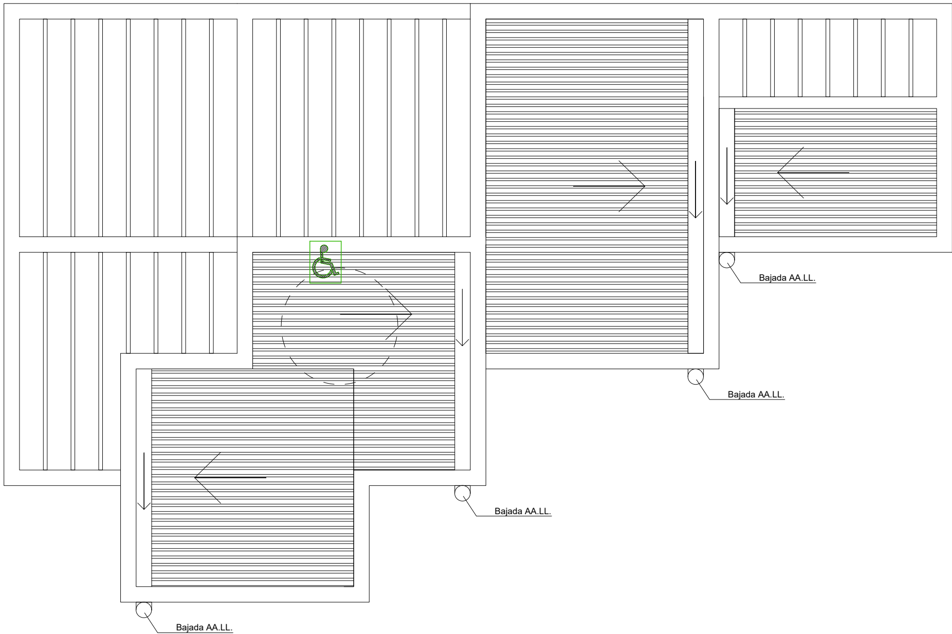
Planta de Cubiertas Kiosco / Enfermeria Esc. 1:50
