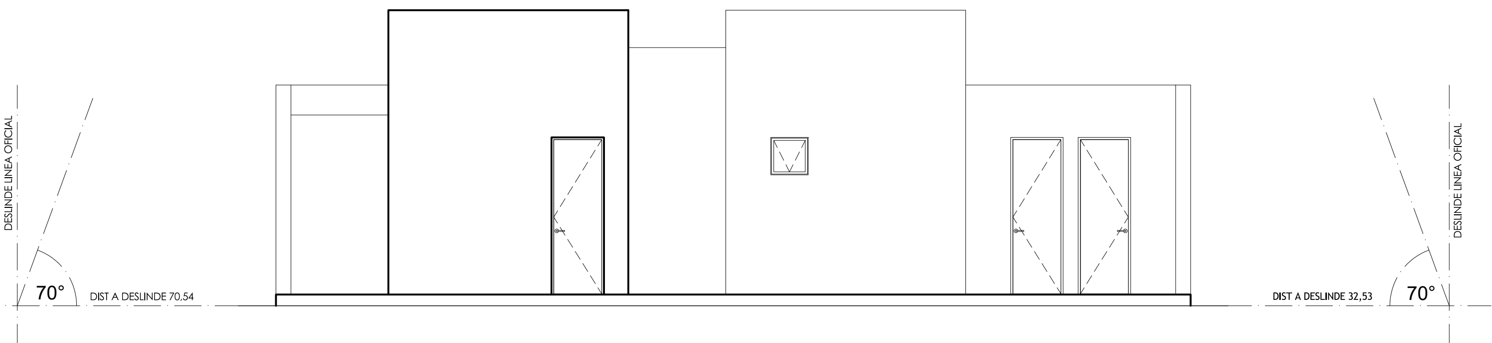
Acceso, Elevación Poniente Esc. 1:50
