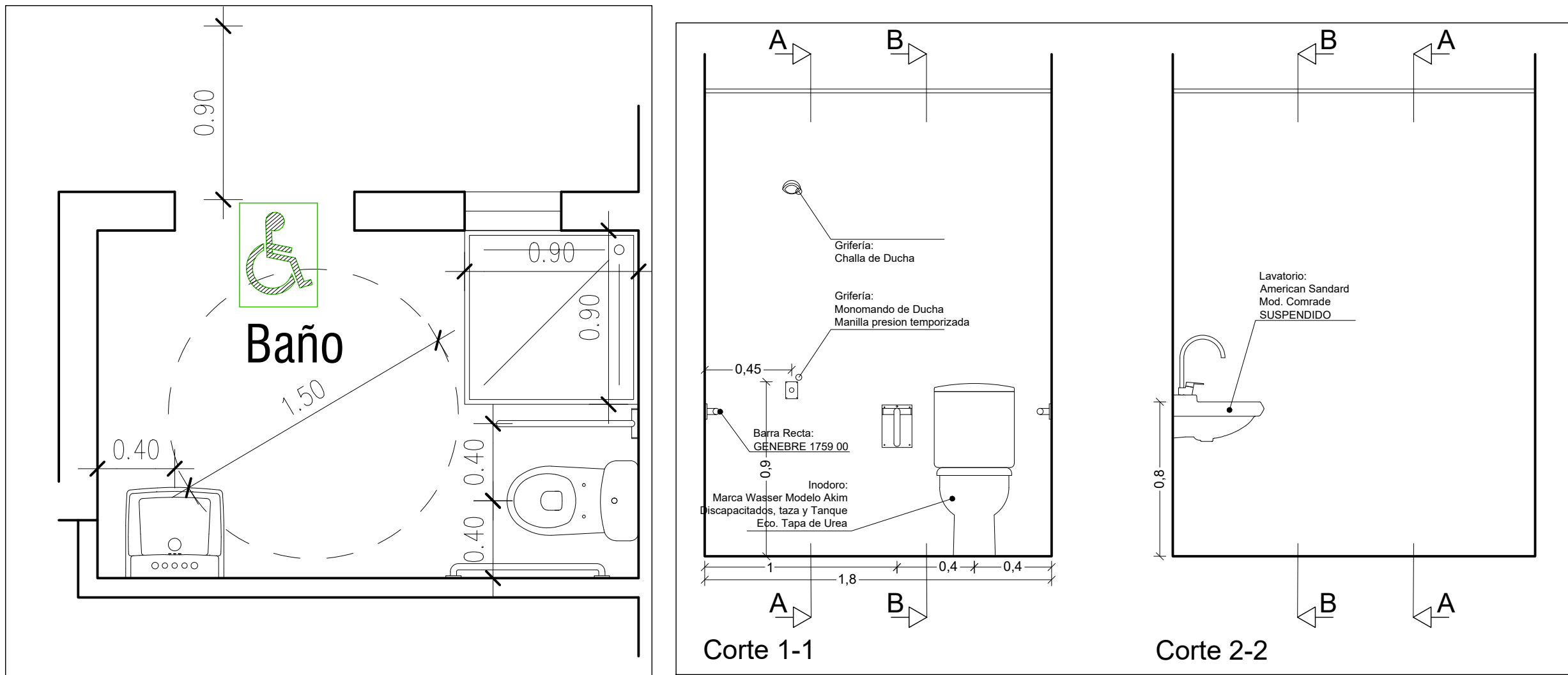
Detalle de baño universal Esc. 1:25
