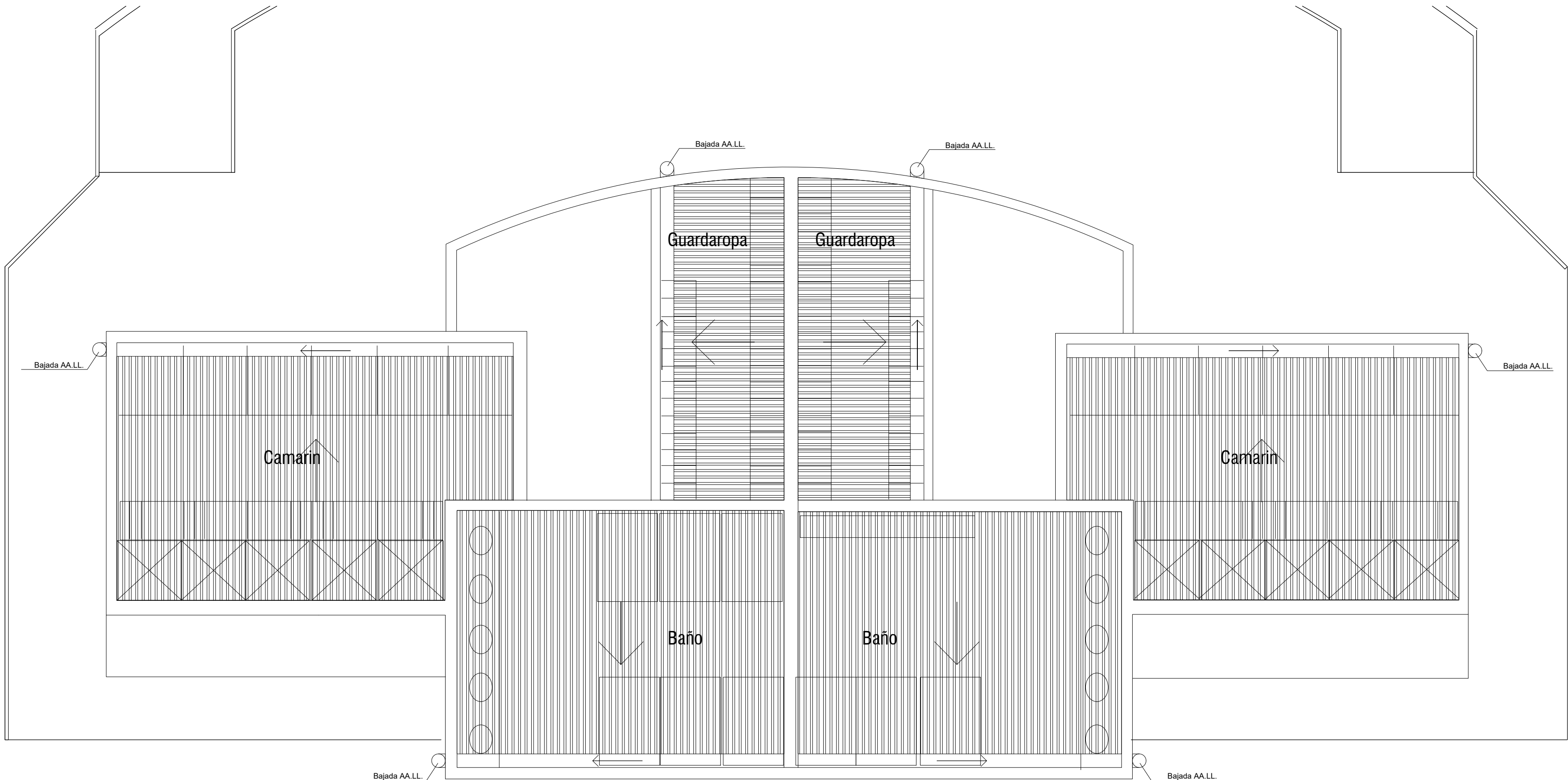
Planta de Cubiertas Acceso Esc. 1:50
