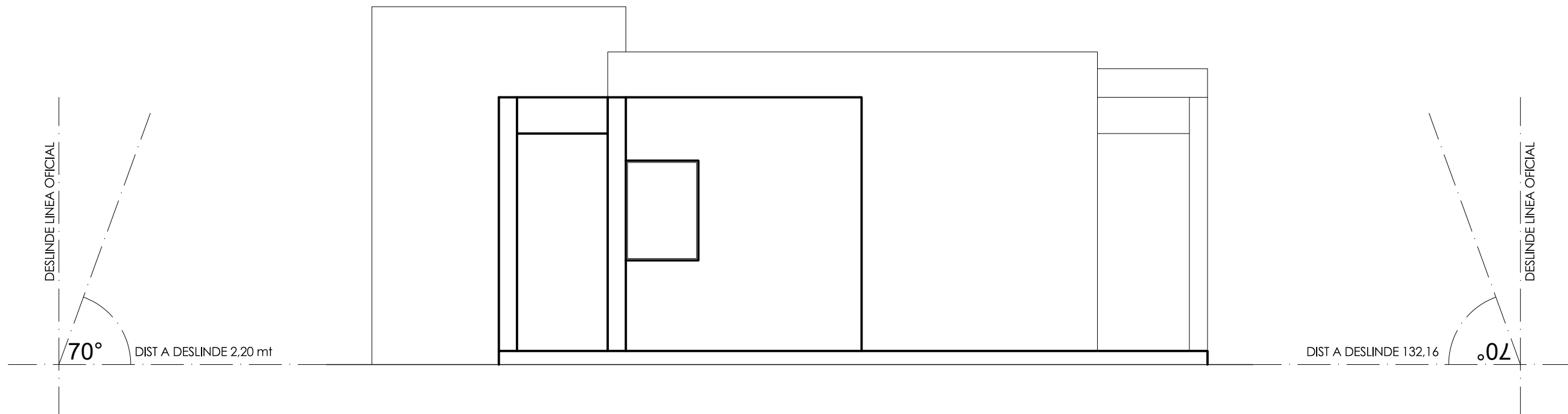
Kiosco / Enfermería, Elevación Sur Esc. 1:50
