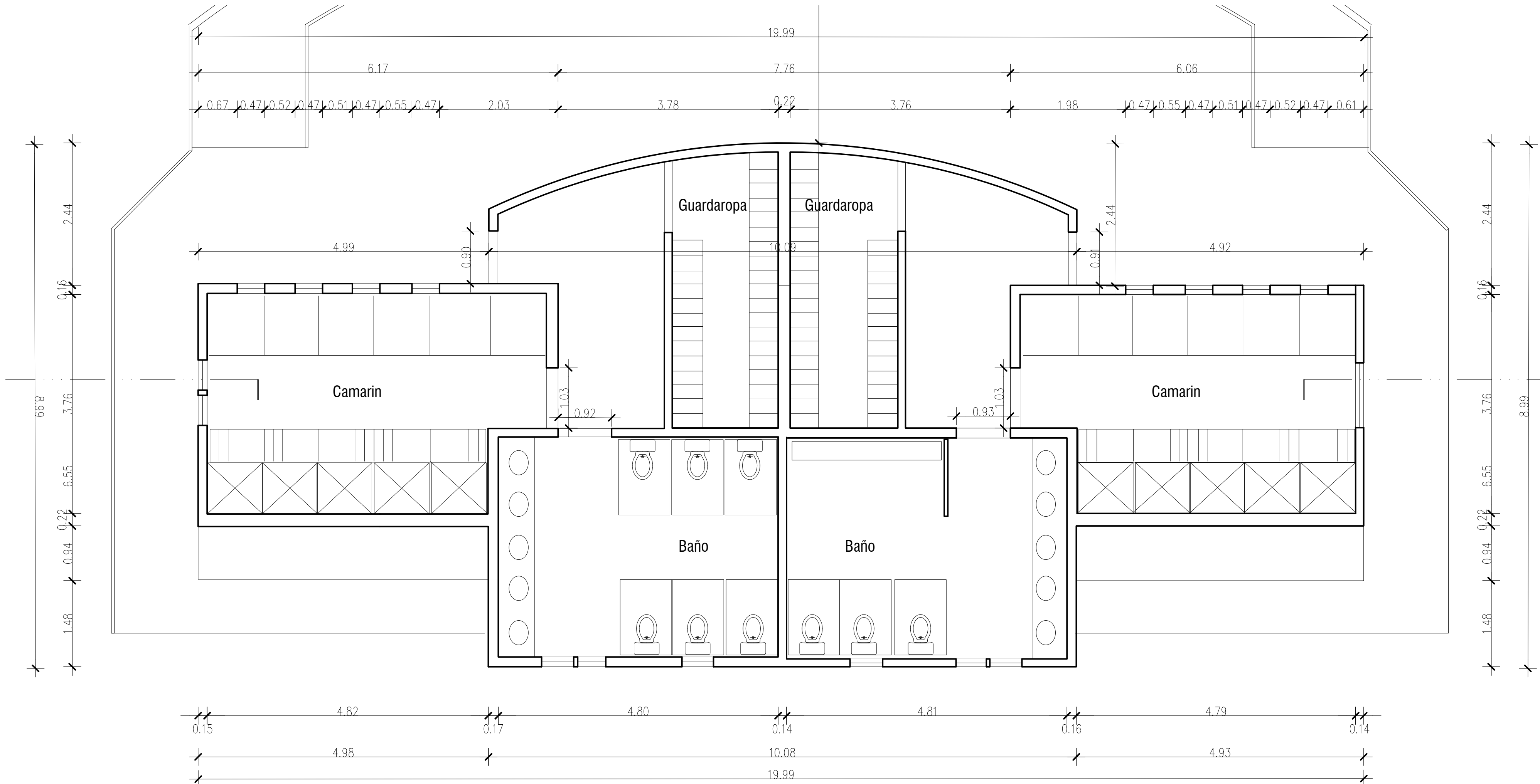
Planta de Camarines Esc. 1:50
