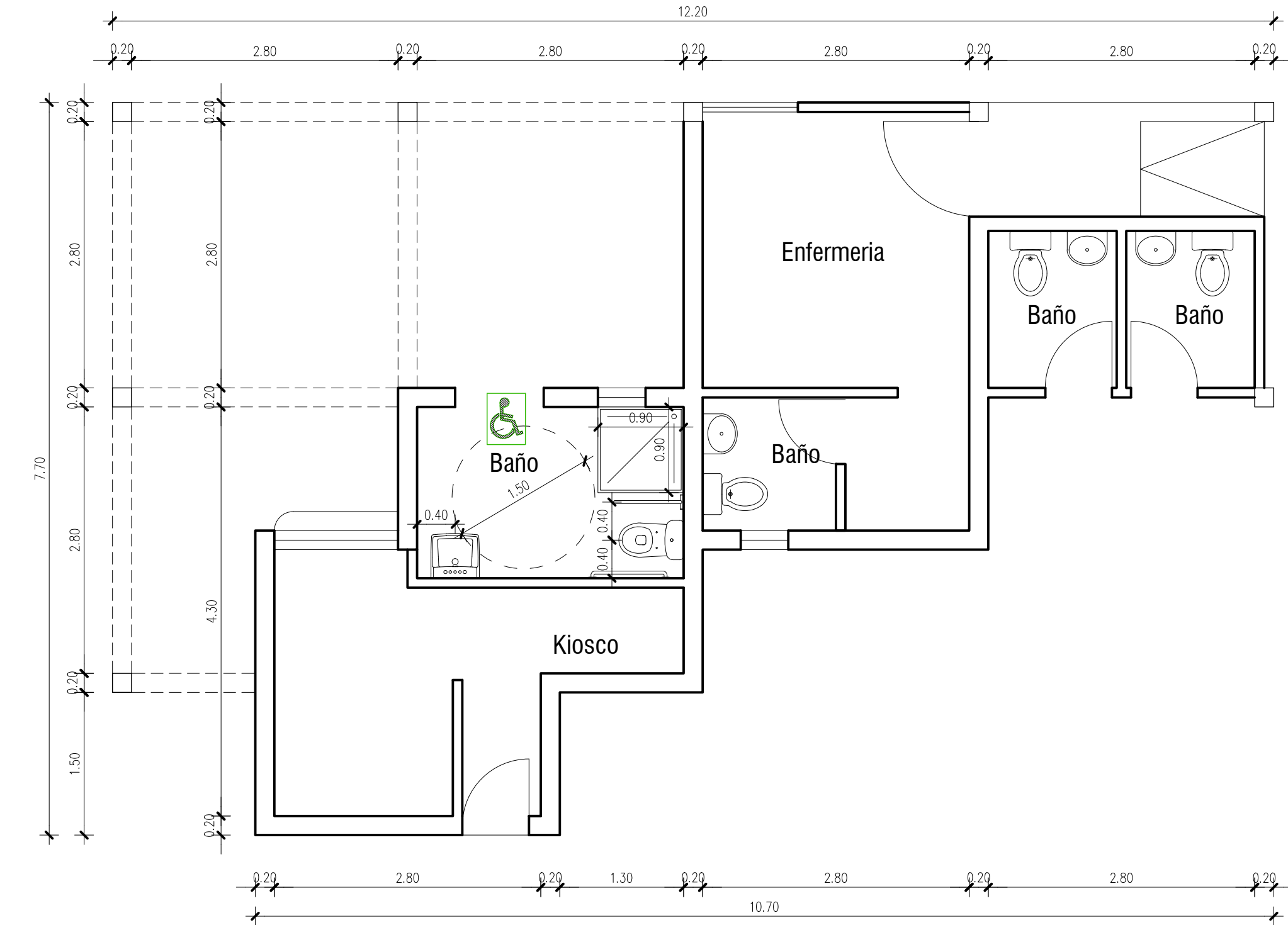
Planta de Kiosco / Enfermeria Esc. 1:50
