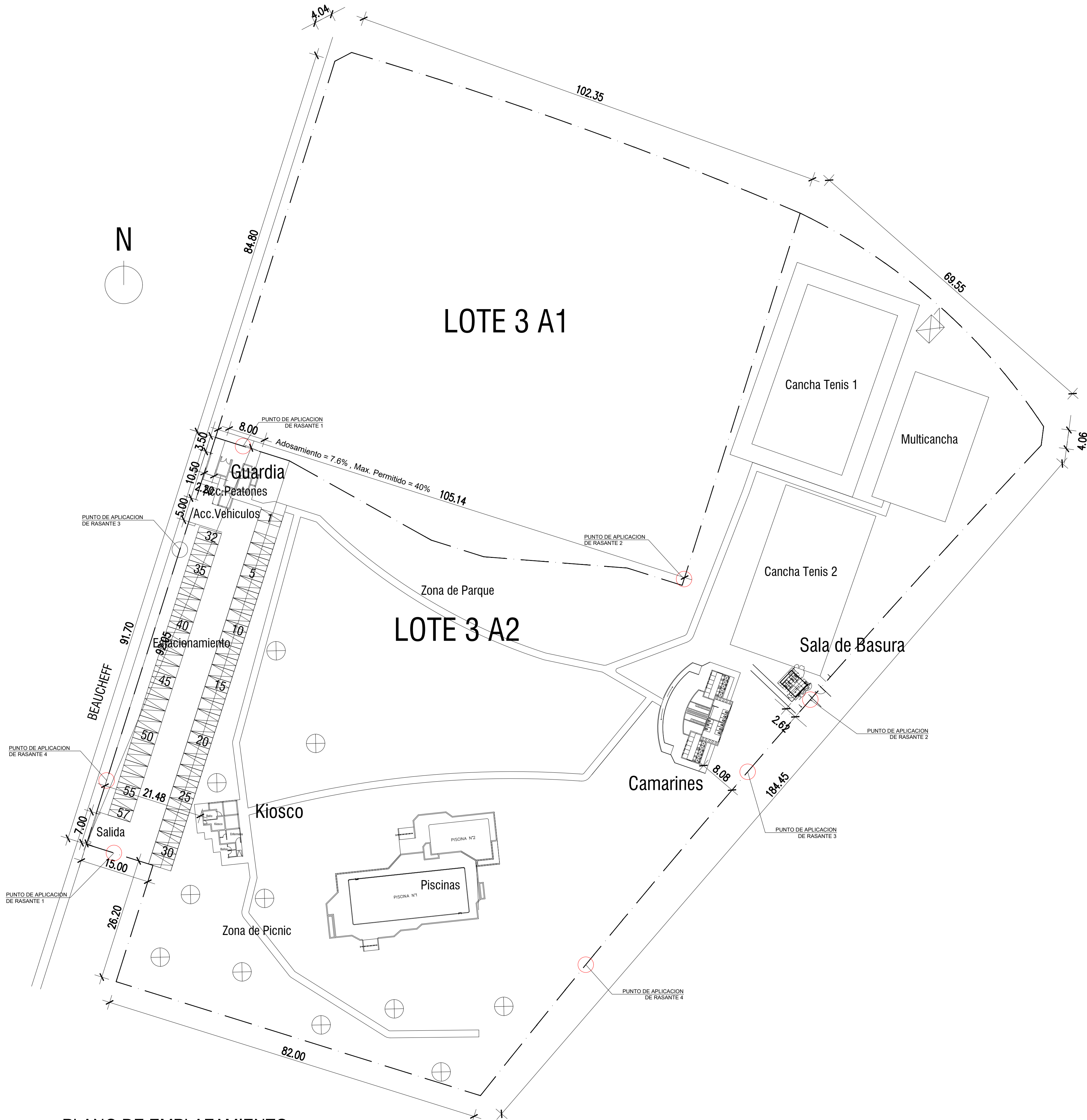
PLANO DE EMPLAZAMIENTO Esc. 1:2000
