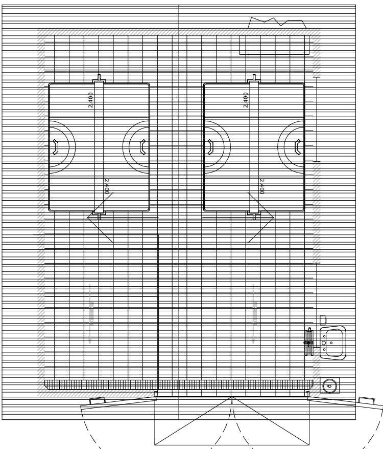
Planta de Cubiertas S. de Basura Esc. 1:50
