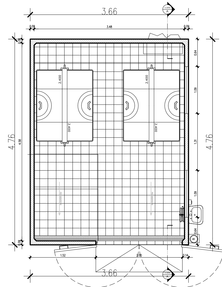
Planta de S. de Basura Esc. 1:50
