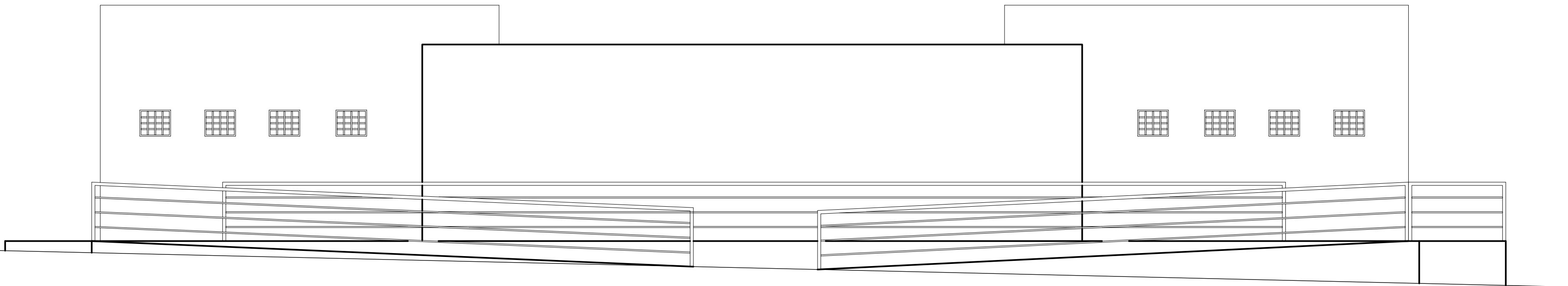
Camarines, Elevación Poniente Esc. 1:500
