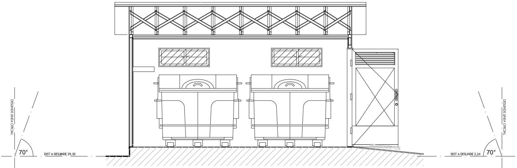
S. Basura, Corte B-B Esc. 1:50
