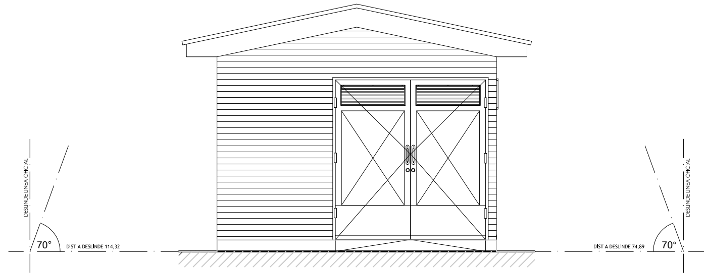
S. Basura, Elevación Oriente Esc. 1:50
