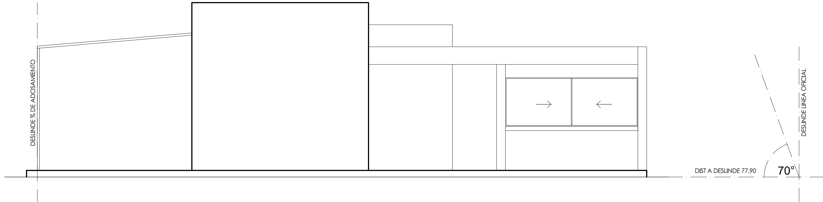
Kiosco / Enfermería, Elevación Poniente Esc. 1:50
