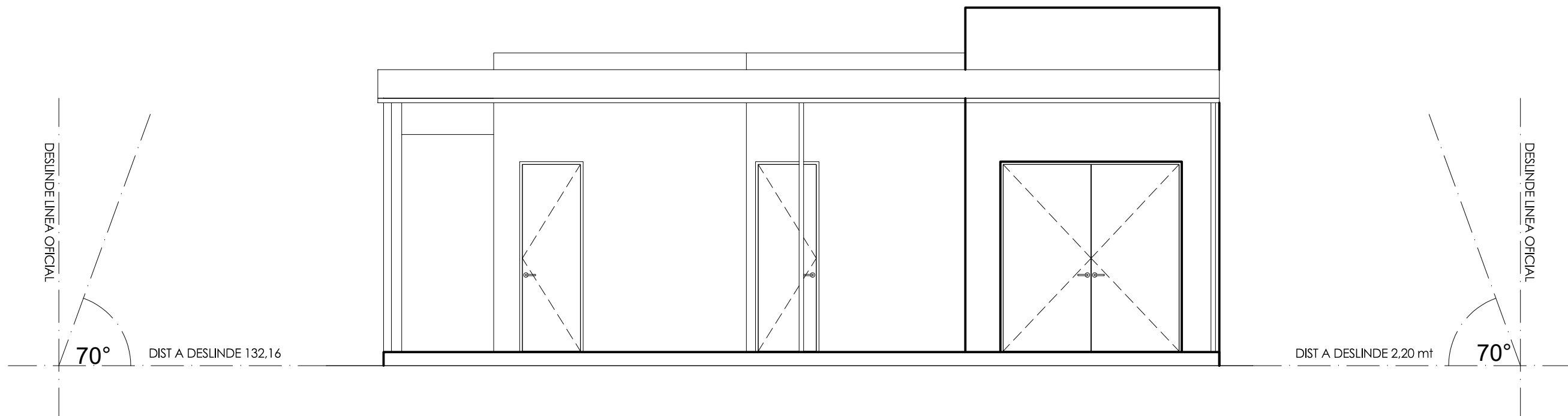
Kiosco / Enfermería, Elevación Norte Esc. 1:50
