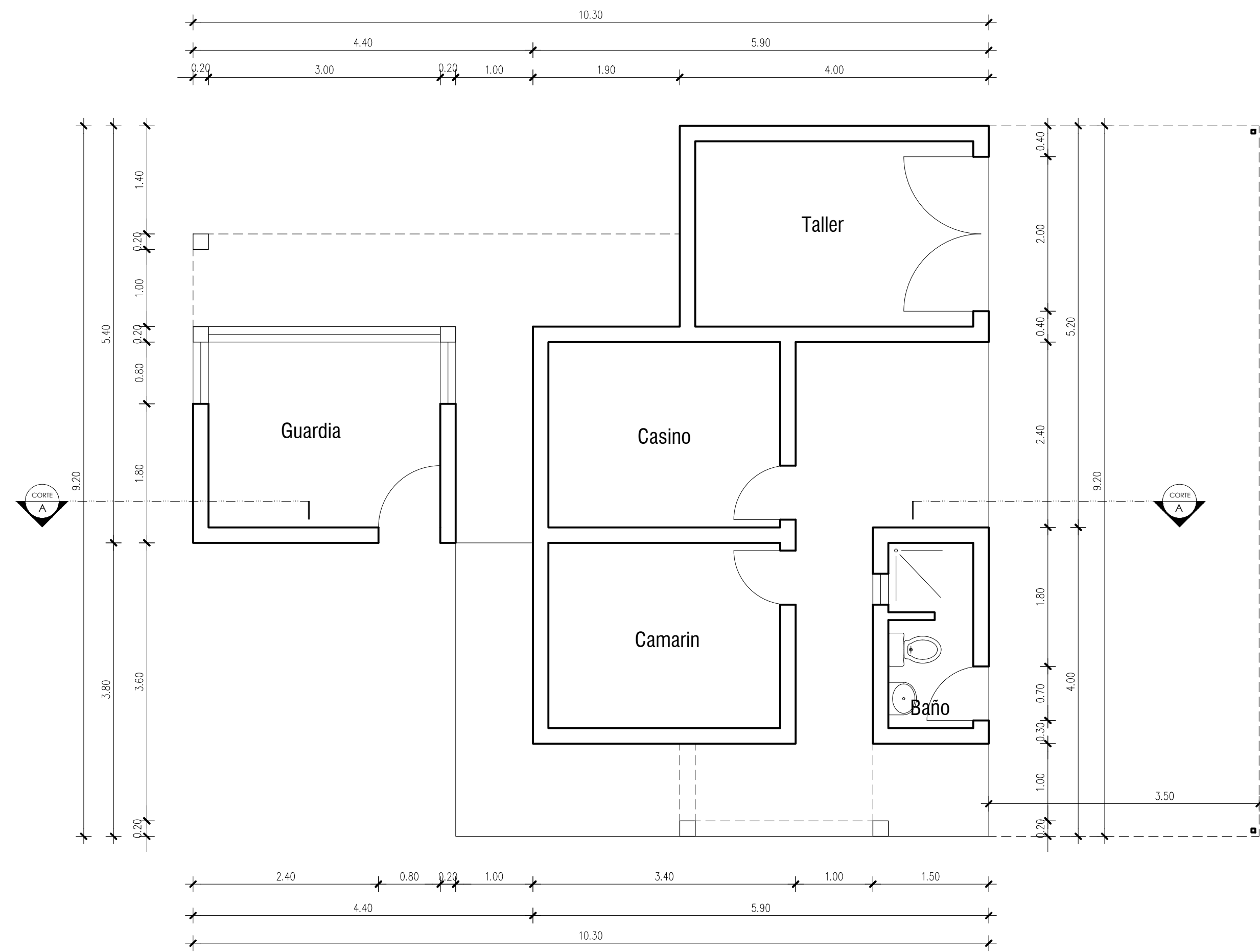
Planta de Acceso Esc. 1:50
